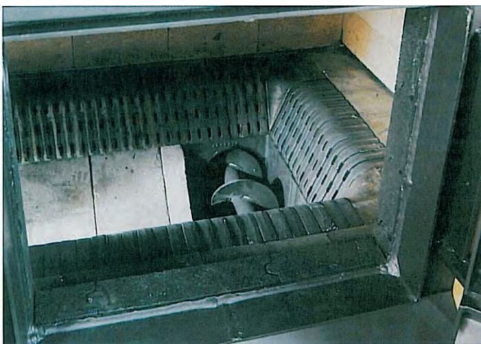
Innenansicht: Schubrechen für Entaschung
